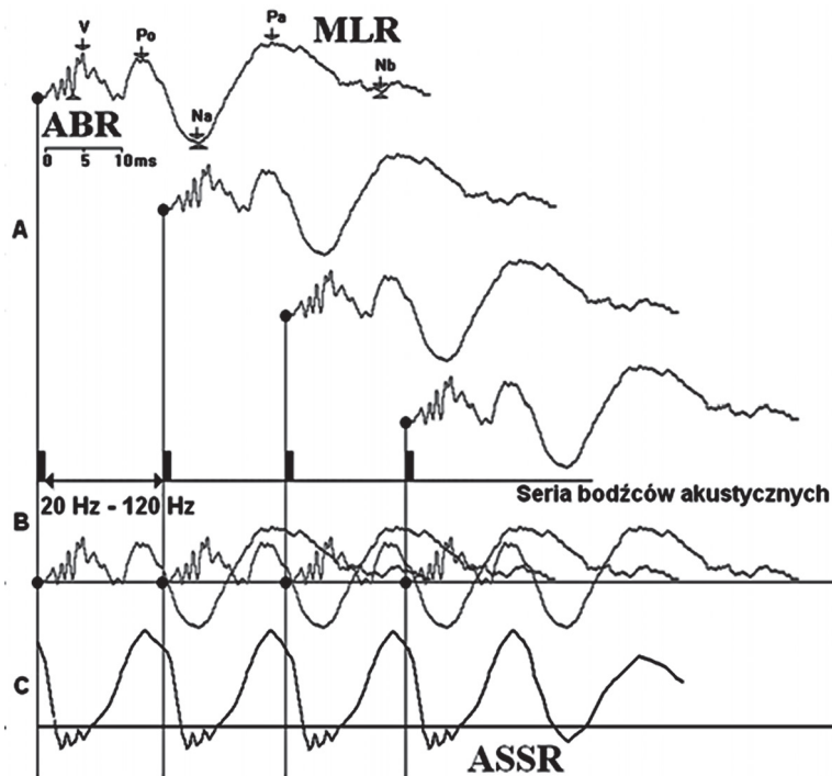
RYSUNEK 11. Schemat usredniania odpowiedzi zapisow czasowych w systemie BioLogic Master 23
