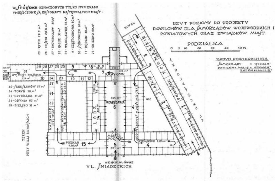
Fot. 9. Plan rozplanowania stoisk w pawilonie samorządowym. Stoiska: 2. województwo śląskie, 16. Królewska Huta, 17. Katowice, 18. Mysłowice, 19. Bielsko, 28. Cieszyn ( Przewodnik po wystawie miast i Związku Miast Polskich . Red. M. POZNAŃSKI. Warszawa 1929)
