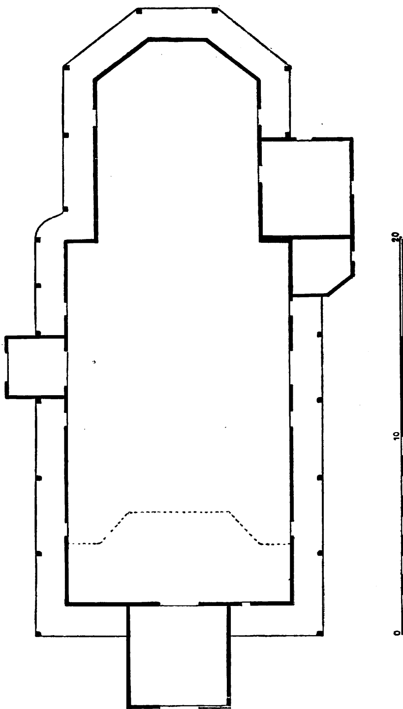
Rzut poziomy kościoła św. Trójcy w Koszęcinie — stan z 1968 r.
